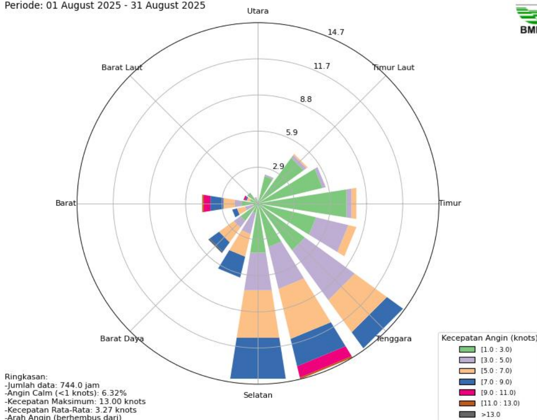
Gambar 7. Kondisi Windrose Bulan Agustus 2025
