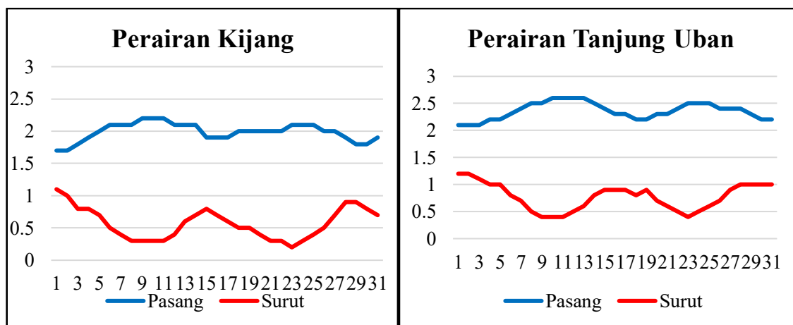
Gambar 8. Analisis Tinggi Pasang - Surut Wilayah Perairan Tanjung Uban dan Kijang Periode Agustus 2025.
