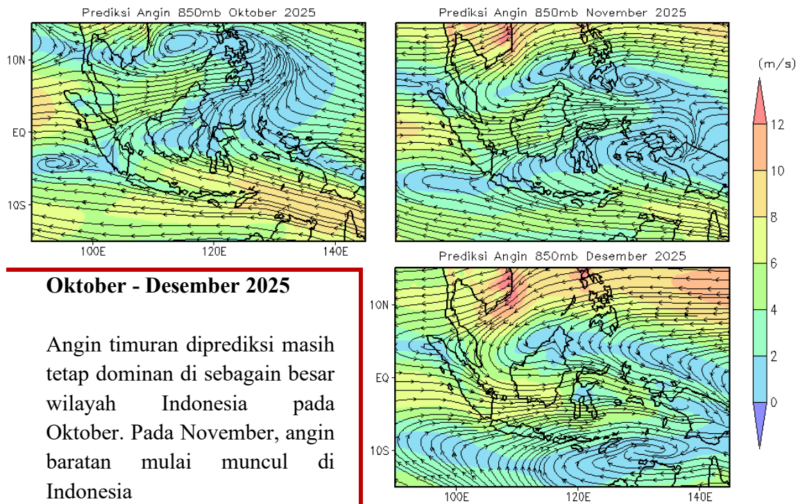
Gambar 6. Prediksi Sirkulasi Angin Bulan Oktober - Desember 2025
